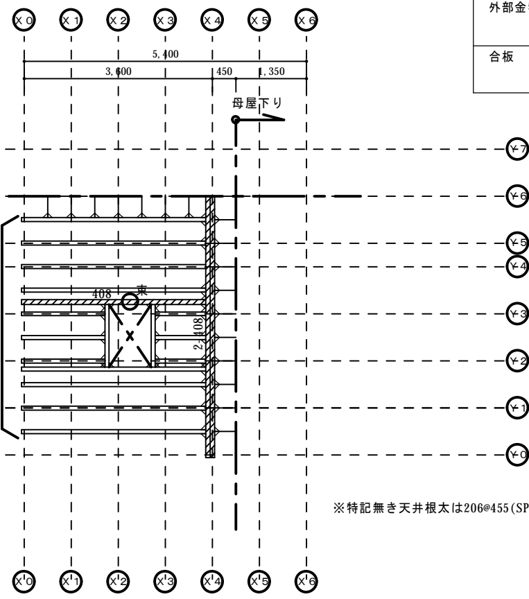
天井伏図 S=1/100
