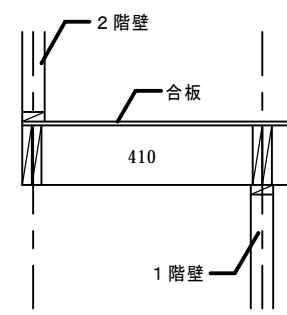
*オーバーハング部分詳細
