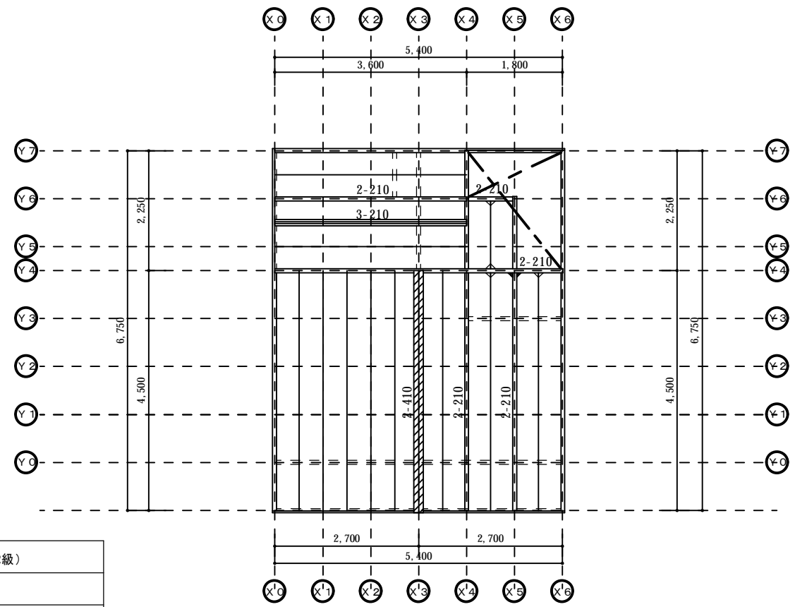
3階床伏図 S=1/100 ※特記無き床根太は210@455(SPF2級)とする
