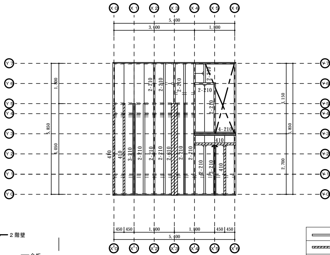
2階床伏図 S=1/100 ※特記無き床根太は210@455(SPF2級)とする
