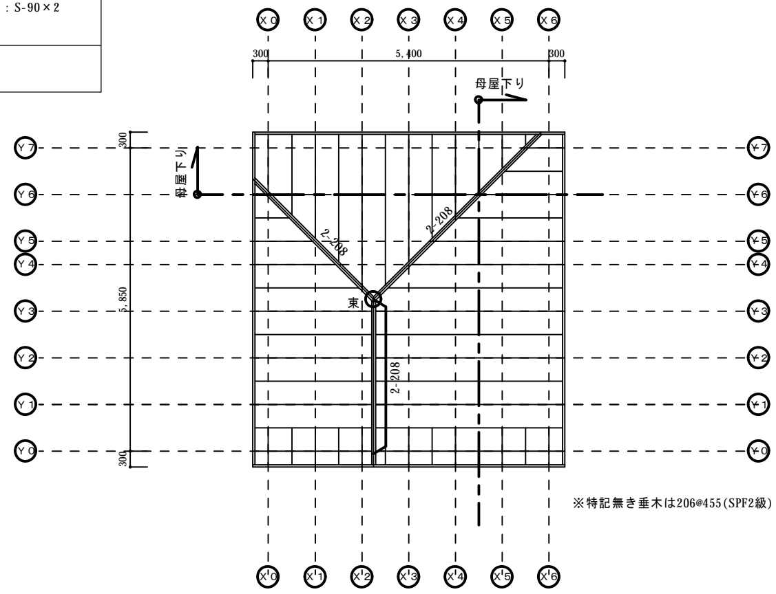
小屋伏図 S=1/100
